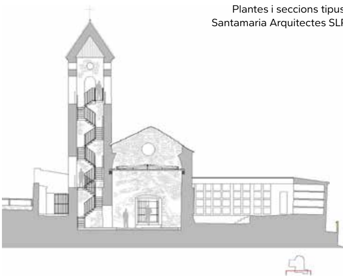
Secció del conjunt. Santamaria Arquitectes SLP
