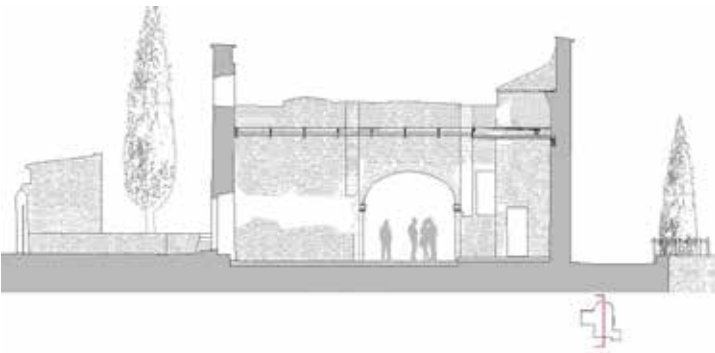
Plantes i seccions tipus. Santamaria Arquitectes SLP
