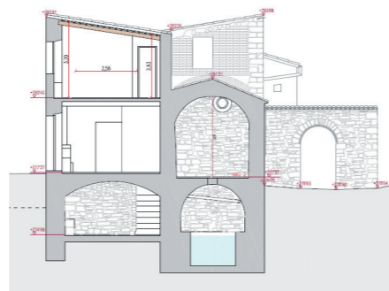
Secció de la Casa de l'ermità i de l'ermita
